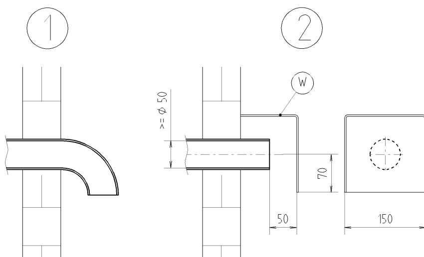
Illustration 3: Vindskydd av tilluftsledning
